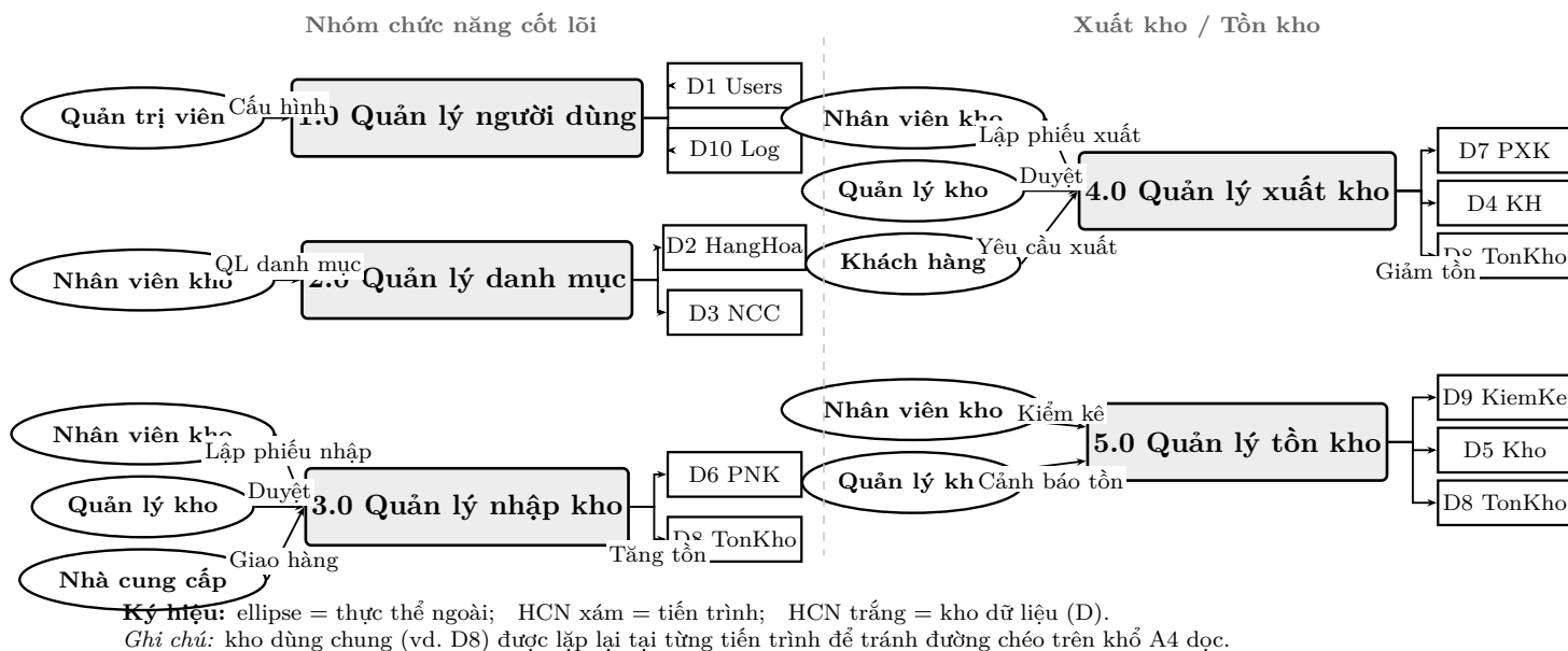
Figure 1: DFD cấp 1 – Phân rã các luồng dữ liệu trong hệ thống quản lý kho hàng
